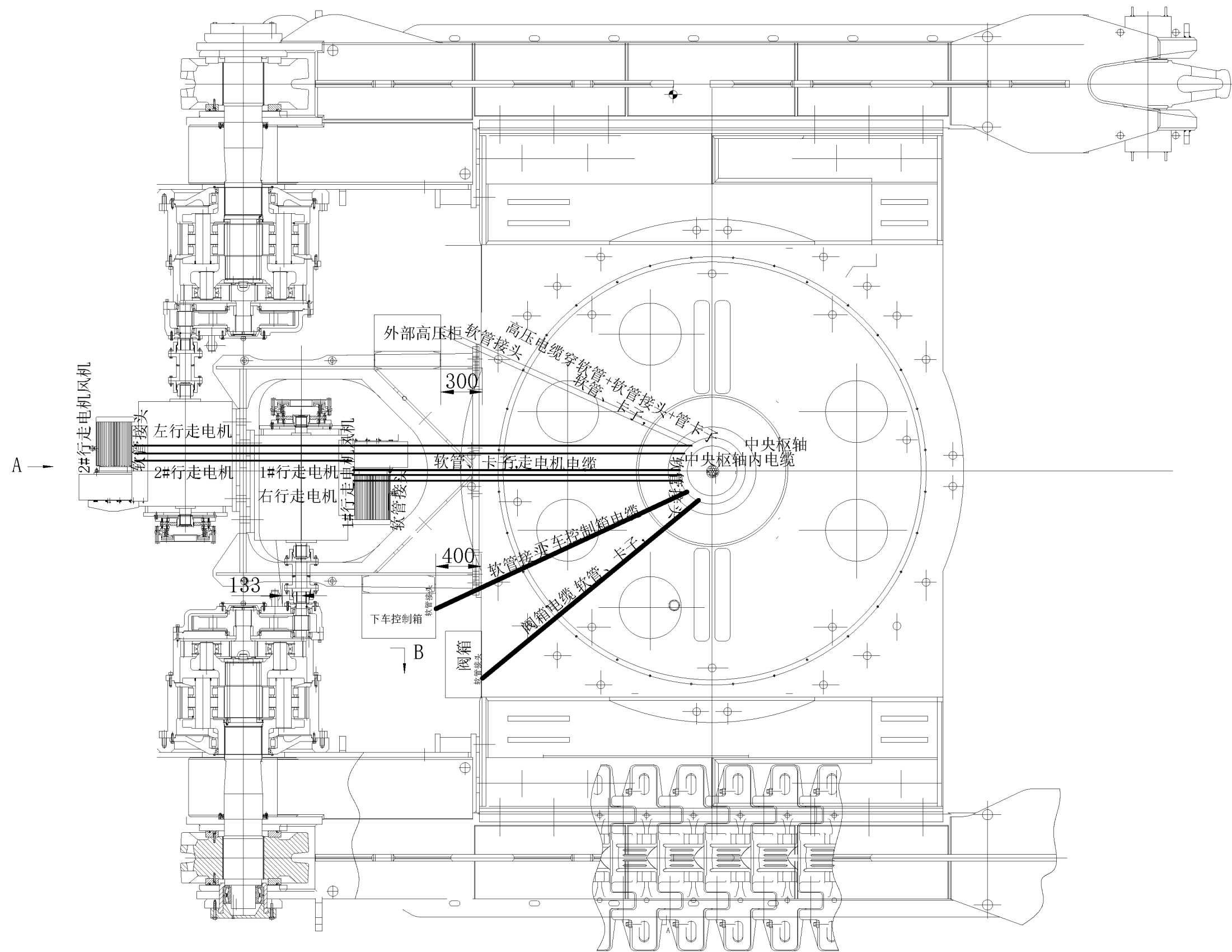
电气下架布置示意图
