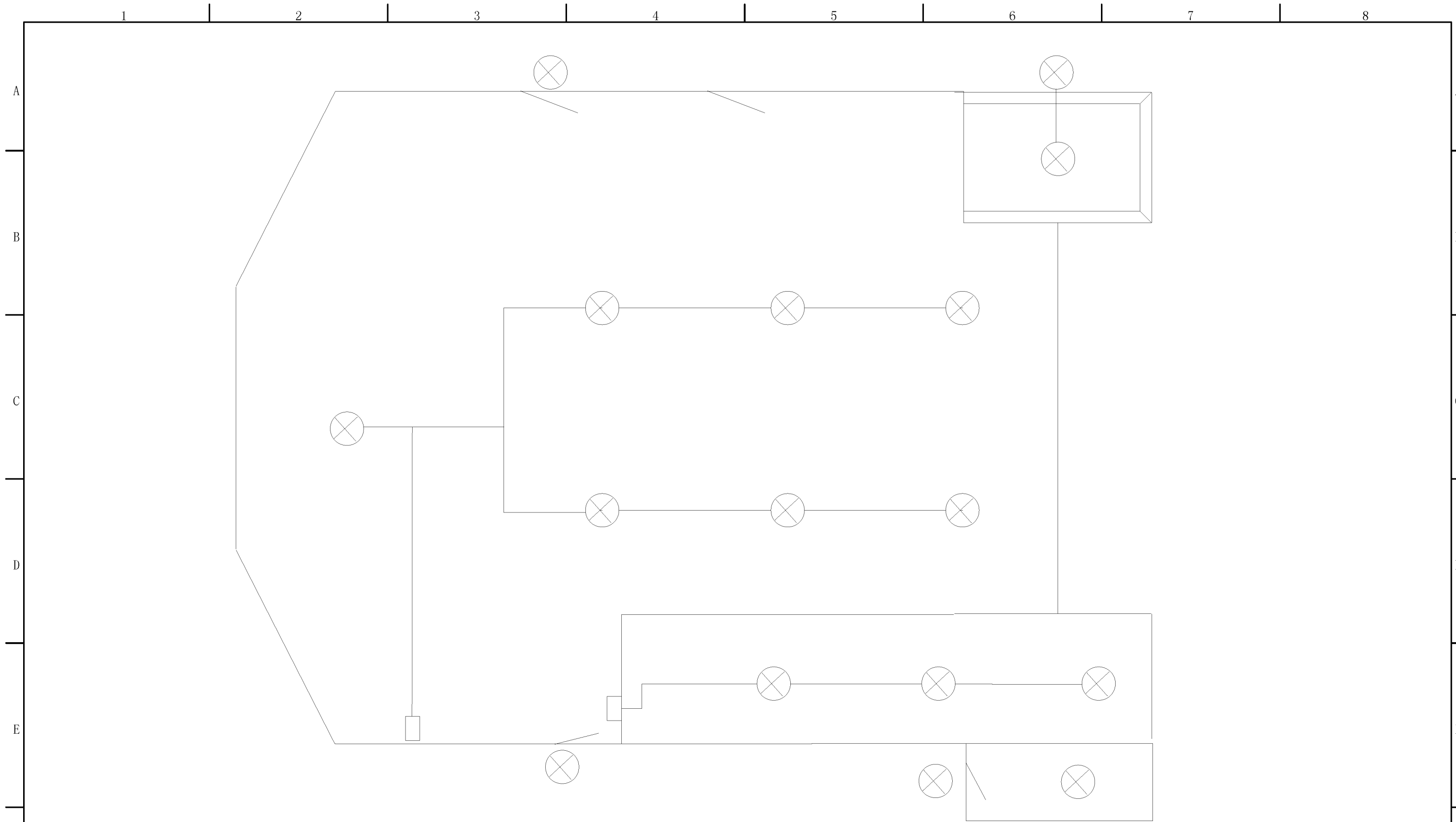
机棚照明示意图
